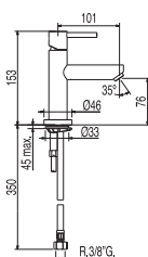
Monomando lavabo Ø 30 mm.
