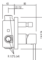
Monomando empotrar baño-ducha
