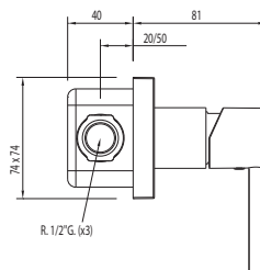
Monomando empotrar ducha
