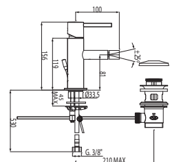
Monomando bidé
